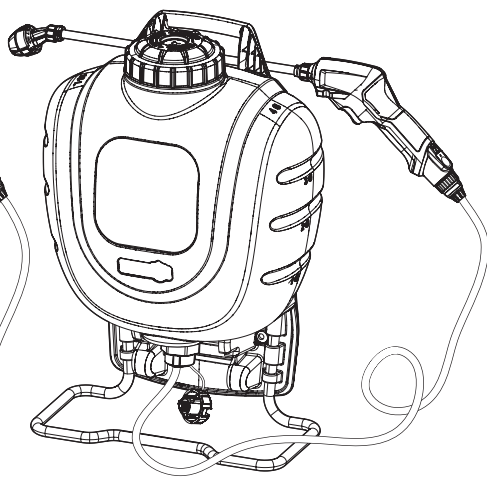
Pulvérisateur à dos de 4 gallons avec lance électrique rechargeable (190802)
